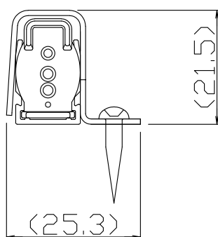
かん合状態
